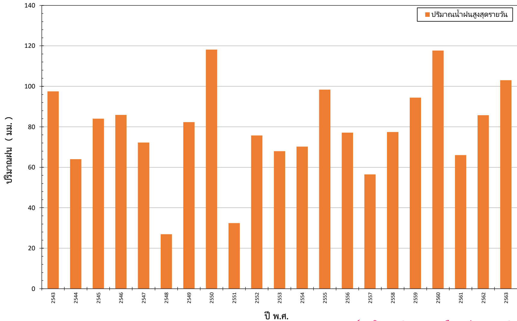
กราฟแสดงปริมาณฝนสูงสุดรายวัน ปีพ.ศ. 2543 - 2563 สถานีน้ำฝน N.8 ( 380111 ) อ.บางมูลนาก จ.พิจิตร
